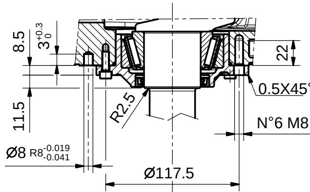
SEZ. A-A
